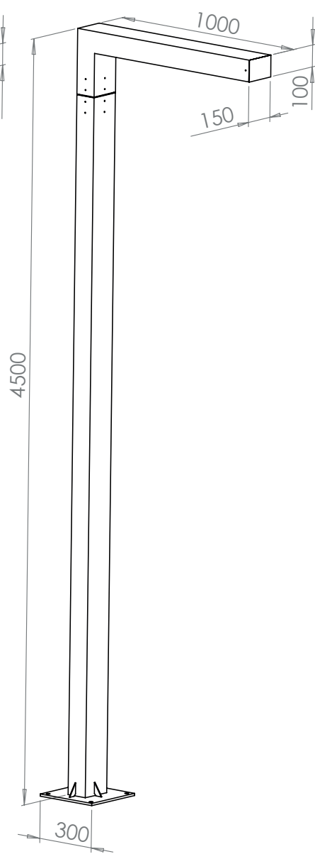
GTM-FN 6-90 4500
