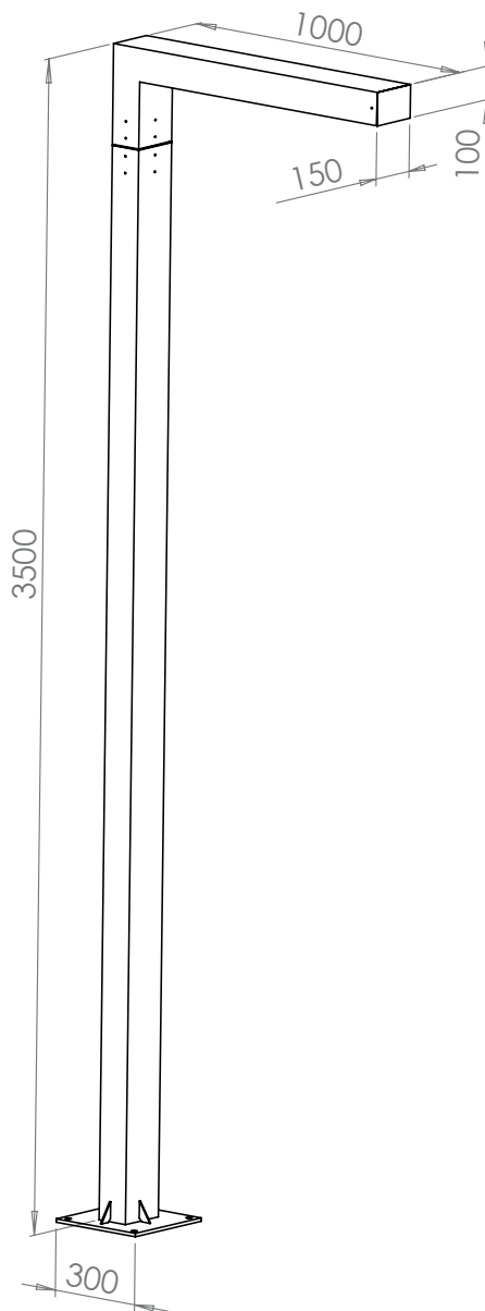
GTM-FN 6-90 3500
