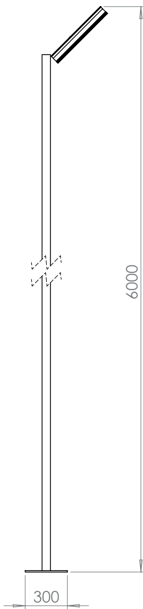
GAL-FN 1-45 6000
